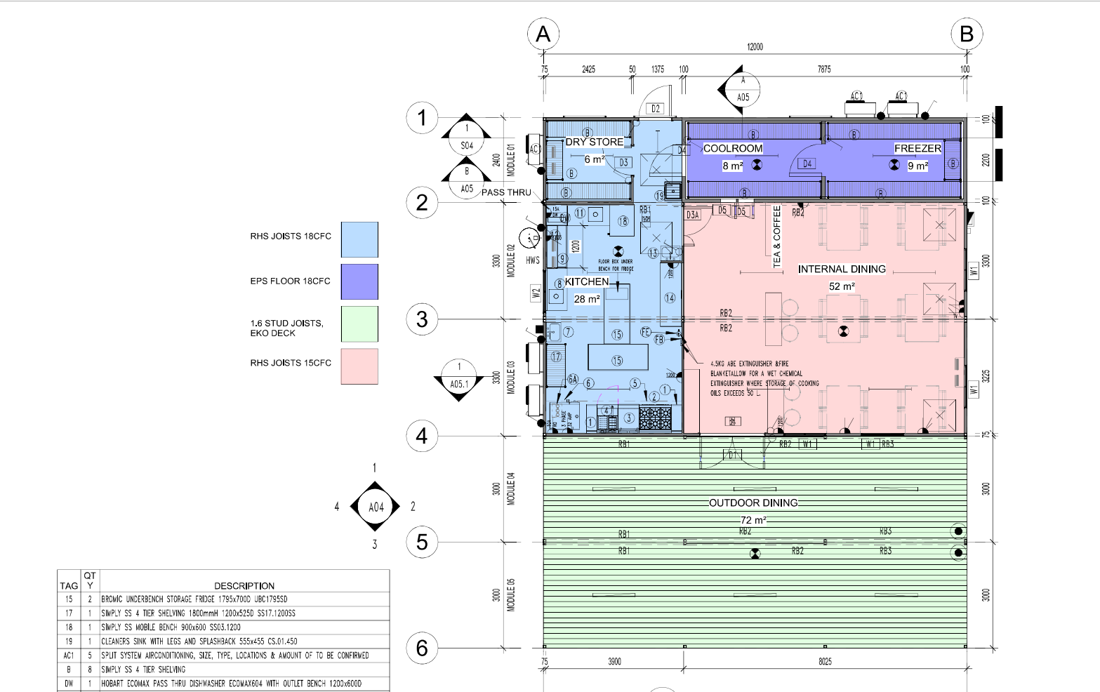
1 A04 FLOOR PLAN 1 : 100
