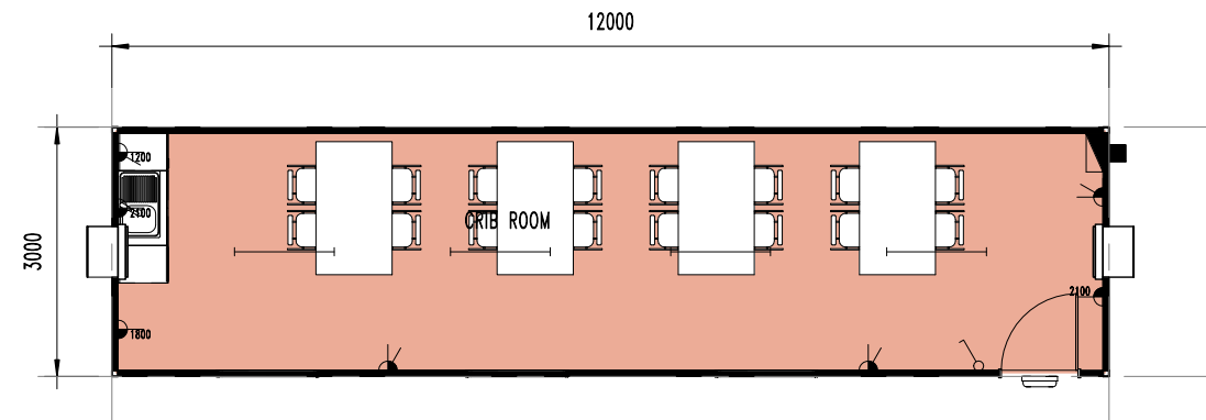
A FLOOR PLAN 1 : 100
